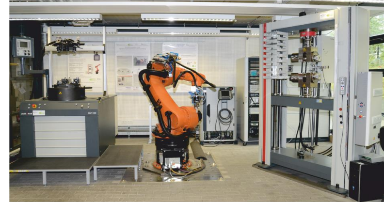
Teleoperative Prüfzelle
